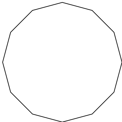
正十二角形
