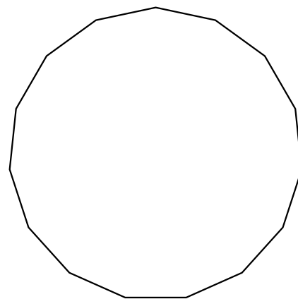
正十五角形
