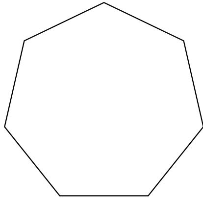
正七角形
