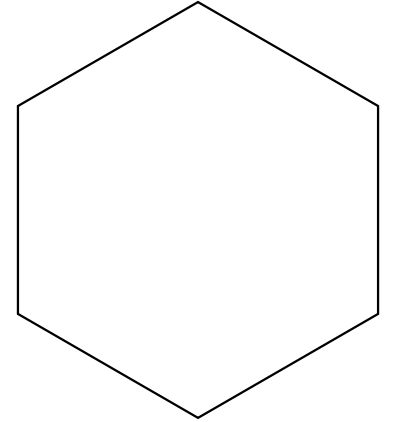
正六角形
