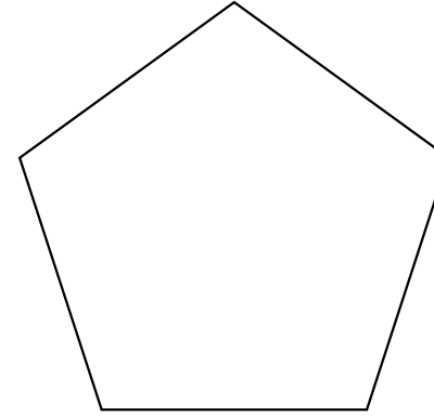
正五角形
