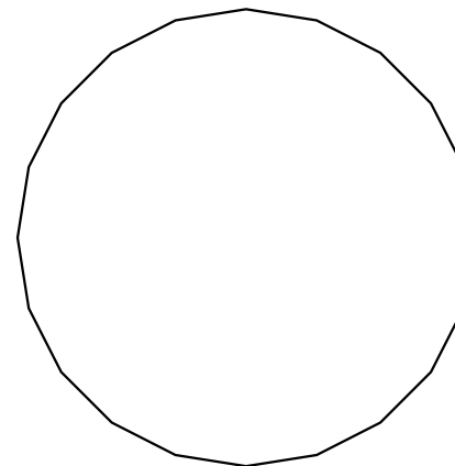
正二十角形
