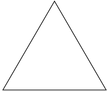
正三角形
