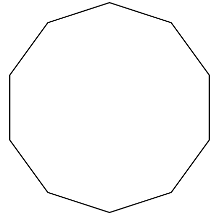
正十角形
