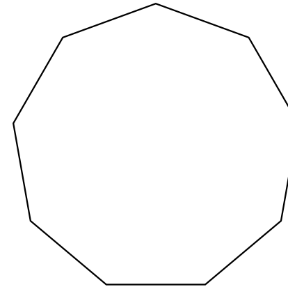
正九角形
