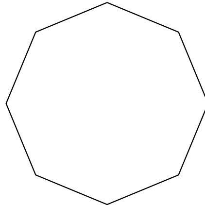
正八角形
